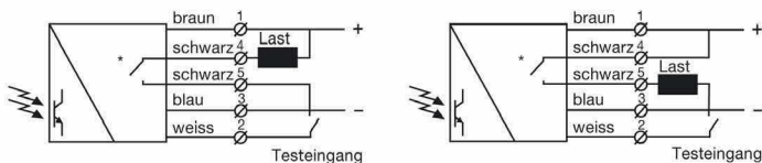
Empfänger SGR 15 mit Halbleiterrelais wird als NPN-Ausgang verwendet
