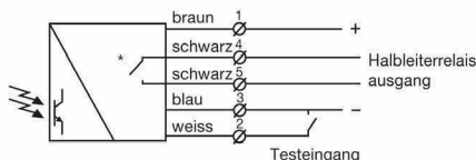
Empfänger SGR 15 mit Halbleiterrelais wird als NPN-Ausgang verwendet
